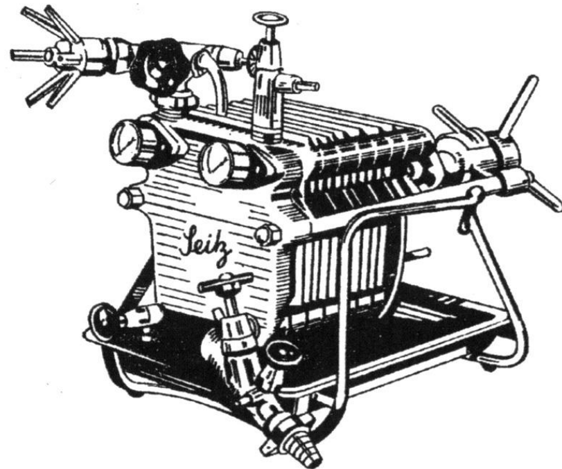
Pilot Z réteges szűrő (Seitz Werke)
